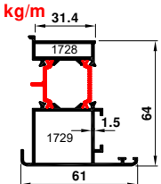
64-1728-1729 1.407 kg/m
