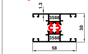
2703 0.403 kg/m
