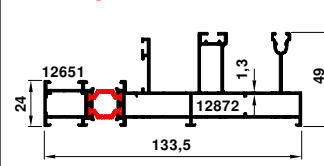
12656 0.351 kg/m
