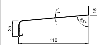
571 0.458 kg/m
