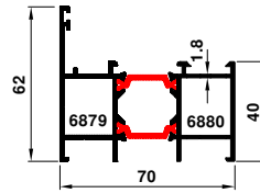
70-7038-7006 1.902 kg/m
