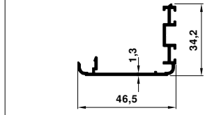
2703 0.403 kg/m
