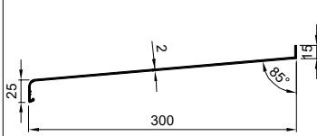
581 1.846 kg/m
