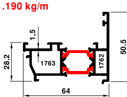
64-1762-1763 1.190 kg/m
