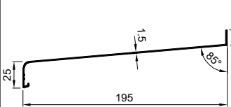
582 0.964 kg/m
