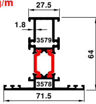
64-1640-1641 1.805 kg/m
