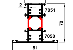
70-7051-7050 2.083 kg/m
