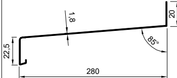
10682 1.587 kg/m
