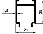
3832 0.175 kg/m
