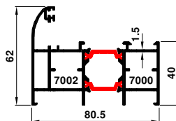
70-8764-12789 2.180 kg/m
