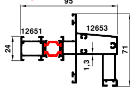
12655 2.435 kg/m
