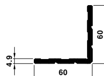
2045 1.436 kg/m
