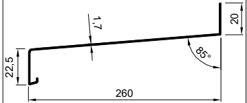
10681 1.408 kg/m
