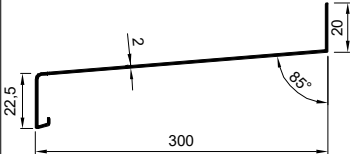
10683 1.868 kg/m
