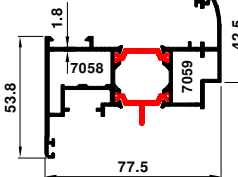
70-7013-7019 2.015 kg/m
