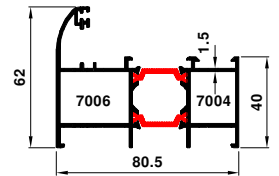
70-7038-7007 2.095 kg/m
