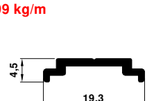
8241 0.099 kg/m
