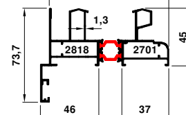
2700-2704-3025 2.700 kg/m
