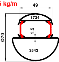
64-1734-3543 1.405 kg/m
