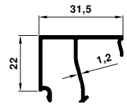
3536 0.329 kg/m
