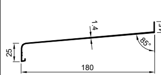
575 0.845 kg/m
