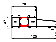
70-7048-7049 1.928 kg/m
