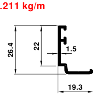
1912 0.211 kg/m
