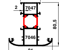
70-7047-7046 2.129 kg/m
