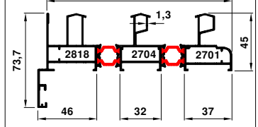
3580-3582 1.902 kg/m
