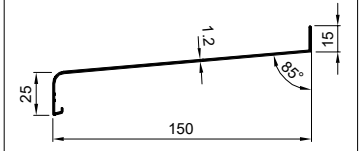
573 0.629 kg/m
