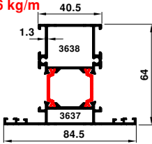
64-1650-1651 1.865 kg/m
