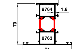
70-8764-8763 1.680 kg/m
