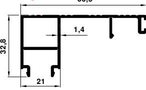
12649 0.666 kg/m
