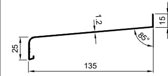
572 0.580 kg/m
