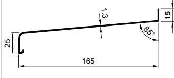
574 0.733 kg/m
